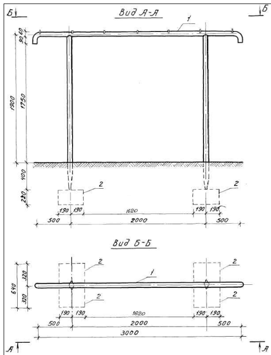
Схема устройства стойки для сушки белья
