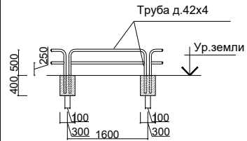
Схема устройства газонного ограждения
