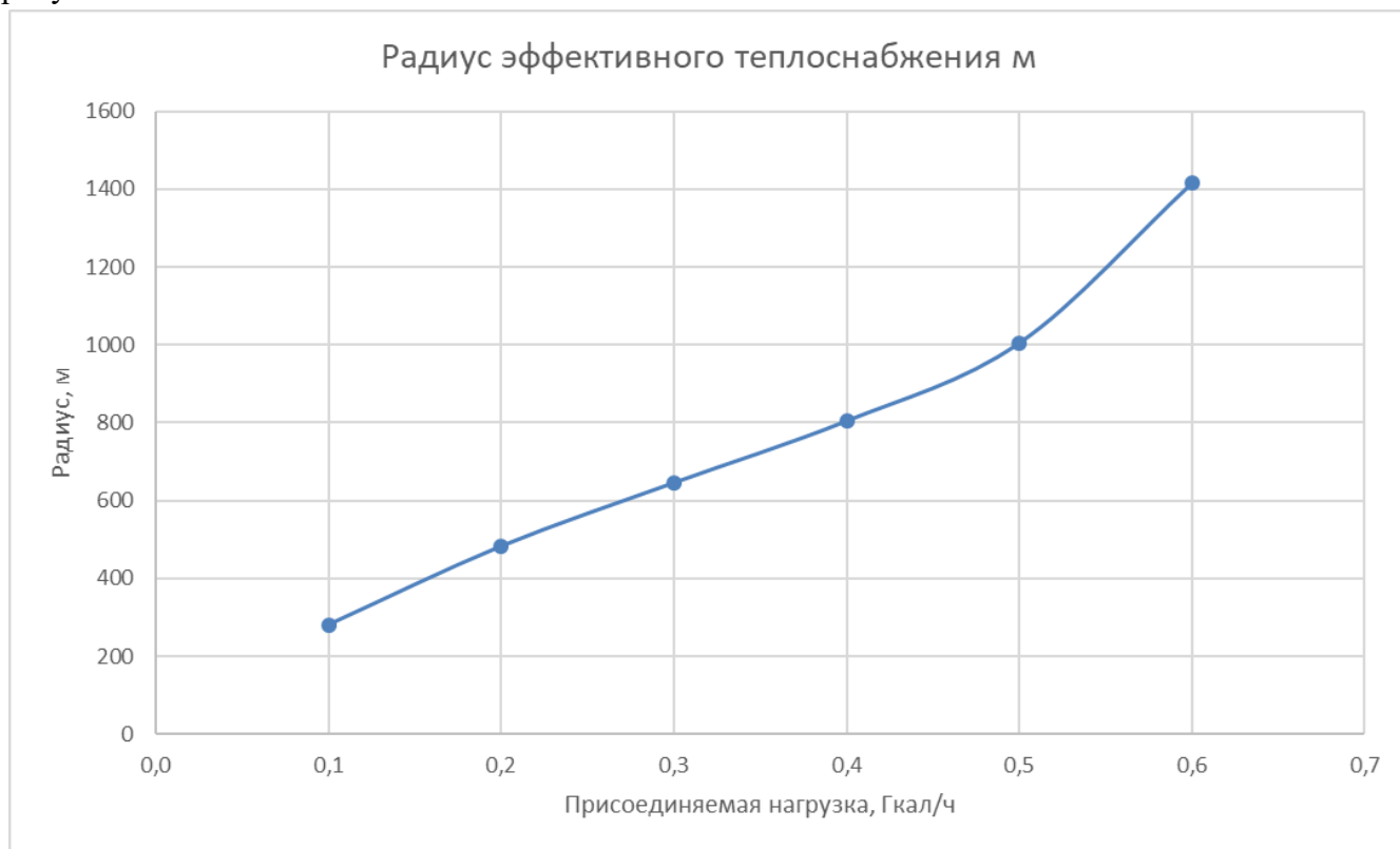
Рисунок 2.3 - Эффективный радиус теплоснабжения, м
