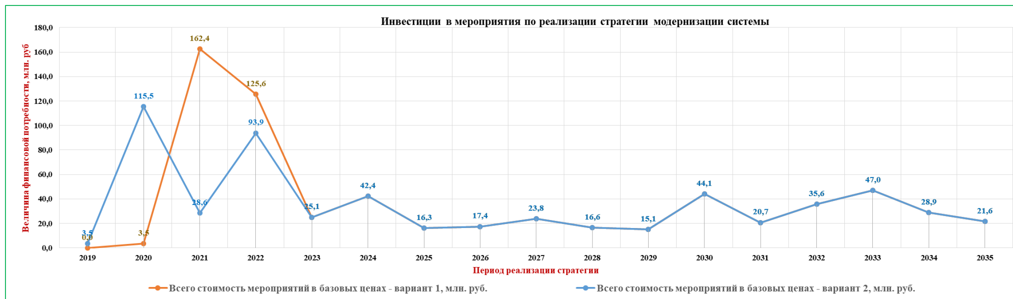
Рисунок 4.1 – Сравнительный график вариантов распределения суммарных инвестиций в реализацию программы развития системы теплоснабжения МО
