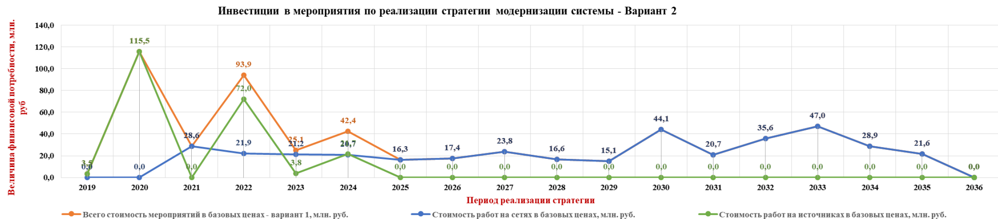
Рисунок 4.3 – Инвестиции в реализацию мероприятий с разбивкой на источники ТЭ и тепловые сети – Вариант 2
