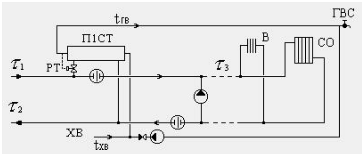
Рисунок 7.1 – Принципиальная схема узла ввода индивидуального теплового пункта
