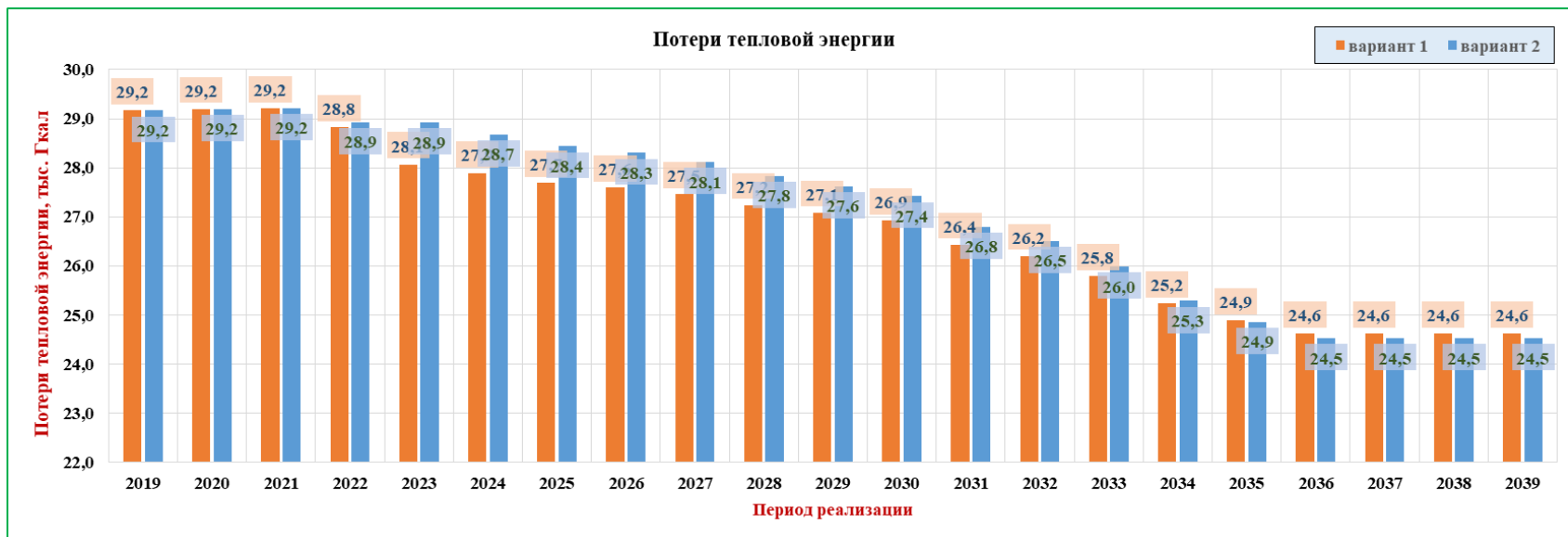
Рисунок 4.7 –Технико-экономическое сравнение вариантов перспективного развития систем теплоснабжения – Потери тепловой энергии
