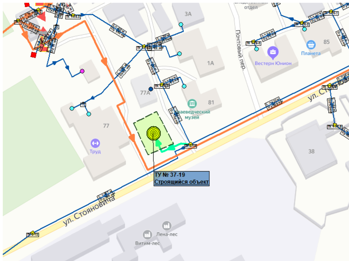
Рисунок 6.7 – Предложения по строительству тепловых сетей для обеспечения перспективных приростов тепловой нагрузки
