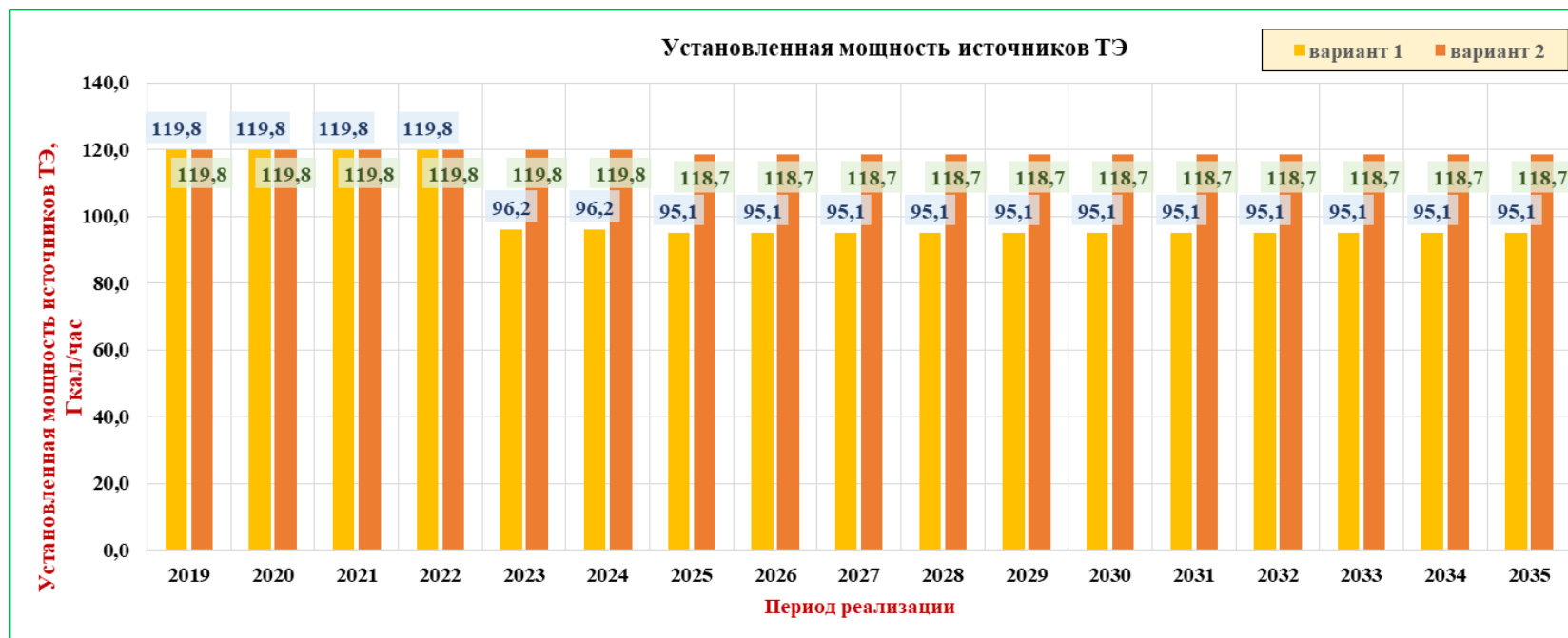
Рисунок 4.4 –Технико-экономическое сравнение вариантов перспективного развития систем теплоснабжения - установленная мощность
