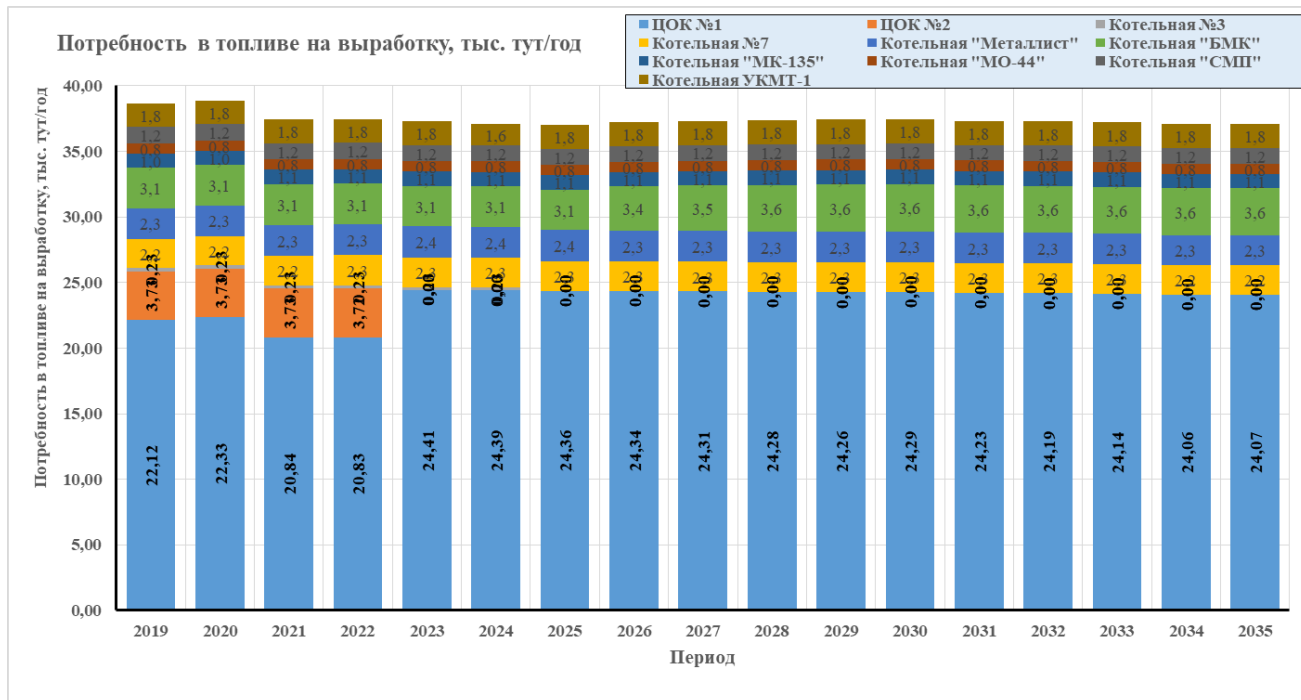
Рисунок 8.1 – Годовой расход условного топлива в разрезе по источнику тепловой энергии
