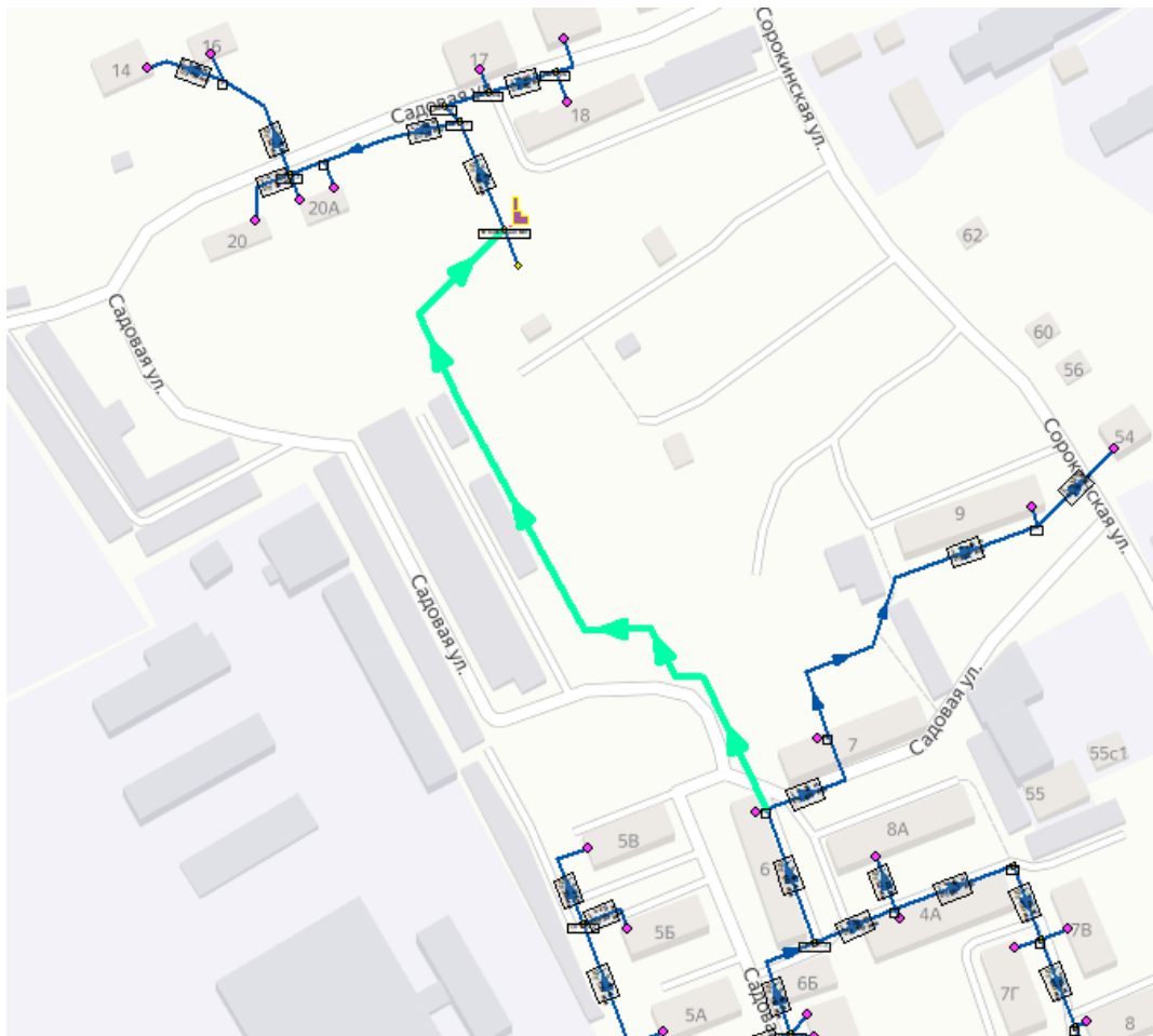
Рисунок 6.1 – Строительство тепловой сети для подключения потребителей котельной №3 к системе котельной УКМТ-1
